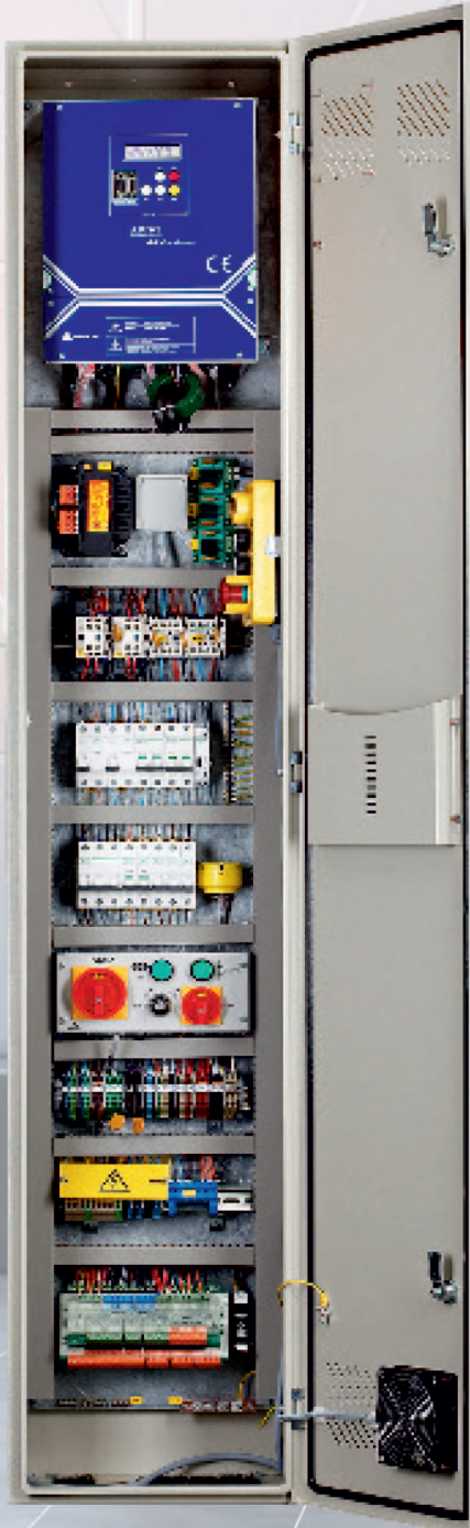
Dişlisiz Pano Gearless Control Panel لوحة التحكم للمحركات بدون تروس
